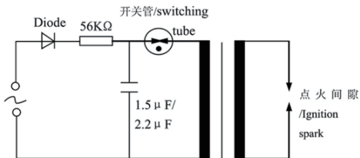
应用电路
